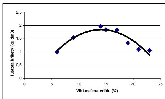
Obr. 1 - Závislosť hustoty brikety od vlhkosti materiálu (drevné piliny). (príklad)
